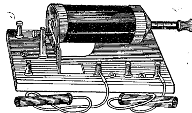
Induktionsapparat N:r 322, stor och kraftig, för primär- och sekundärström, monterad å valnötsplatta, med 2 handtag och ledningssnören. Pr st. .... Kr. 6.25
