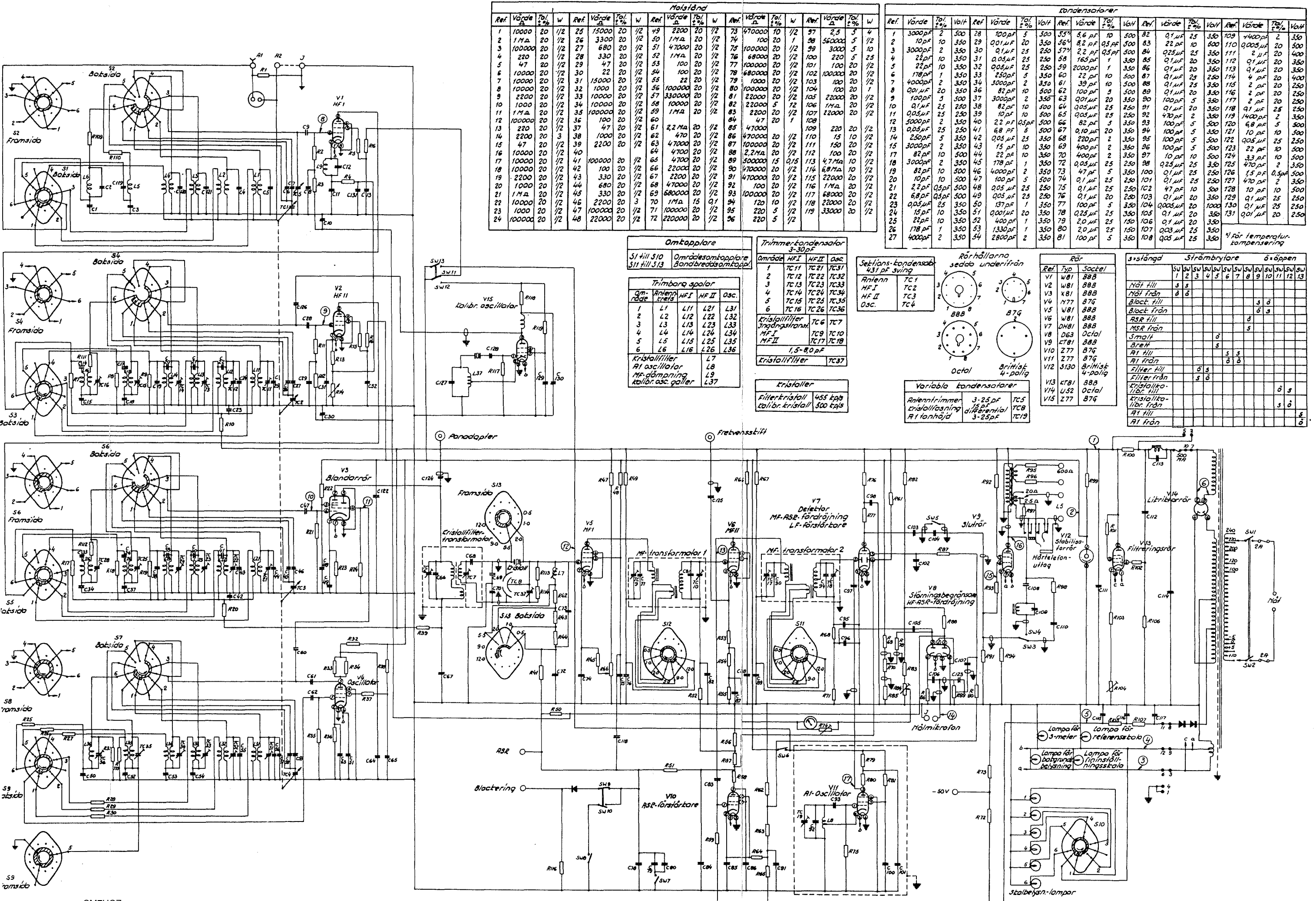
BILD 14 KRETSSCHEMA FÖR KV-MOTTAGARE m/50 Ritning F1107-108651-1
